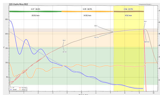
Figure 24. An actual roast log
